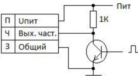
Схема выходного частотного каскада блока "АВ-2Р-А"
